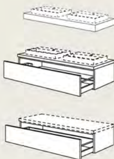
120 cm Doppelwaschtisch
